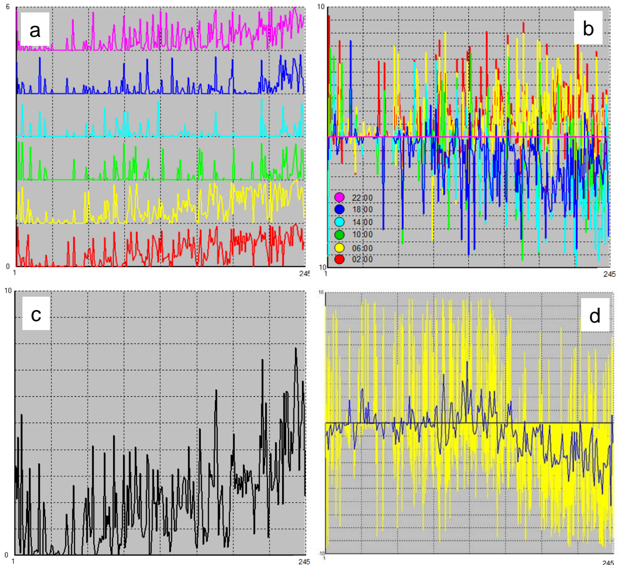
Abb. 3: Verschiedene Darstellungsformen der Blattnässe (in %) für den Zeitbereich 01.03.2020 bis 31.10.2020. Präsentiert ist der Mittelwert über alle Stationen. Abb. 3a: Blattnässe zu verschiedenen Tageszeiten. Abb. 3b: wie 3a, wobei allerdings die Abweichung von der Blattnässe um 22 Uhr gezeigt wird. Abb. 3c stellt die mittlere Blattnässe dar und Abb. 3d die Abweichung der mittleren Blattnässe gemessen bei Großhöflein, dem trockensten Standort, vom Mittelwert aller Standorte (blaue Linie). Gelb ist die Abweichung für jeden Messzeitpunkt (96 pro Tag) vom Mittelwert aller Standorte dargestellt.
