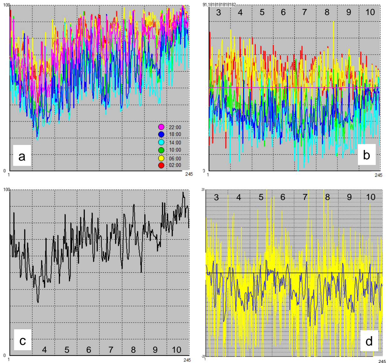
Abb. 2: Verschiedene Darstellungsformen der Relativen Luftfeuchte (in %) für den Zeitbereich 01.03.2020 bis 31.10.2020. Präsentiert ist der Mittelwert über alle Stationen. Abb. 2a: Relative Luftfeuchte zu verschiedenen Tageszeiten. Abb. 2b: wie 2a, wobei allerdings die Abweichung von der Luftfeuchte um 22 Uhr gezeigt wird. Abb. 2c stellt die mittlere Relative Luftfeuchte dar und Abb. 2d die Abweichung der mittleren Relativen Luftfeuchte am Standort Jois, dem trockensten Ort, vom Mittelwert aller Standorte (blaue Linie). Gelb ist die Abweichung für jeden Messzeitpunkt (96 pro Tag) vom Mittelwert aller Standorte dargestellt.
