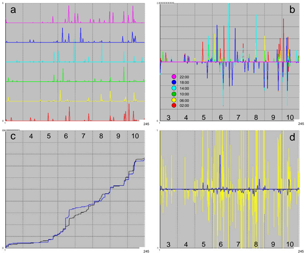
Abb. 4: Verschiedene Darstellungsformen des Niederschlags (in mm) für den Zeitbereich 01.03.2020 bis 31.10.2020. Präsentiert ist der Mittelwert über alle Stationen in Abb. 4a und 4b. Abb. 4a: Niederschlag zu verschiedenen Tageszeiten. Abb. 4b: wie 4a, wobei allerdings die Abweichung von der Niederschlagsmenge um 22 Uhr gezeigt wird. Abb. 3c stellt den mittleren, kumulativen Niederschlagsverlauf im Zeitintervall dar (schwarz) und zum Vergleich den Verlauf am Standort Edelstal (blau). Abb. 4d stellt die Abweichung des Niederschlags in Edelstal vom Mittelwert aller Stationen dar (blaue Linie). Gelb ist die Abweichung für jeden Messzeitpunkt (96 pro Tag) vom Mittelwert aller Standorte präsentiert.
