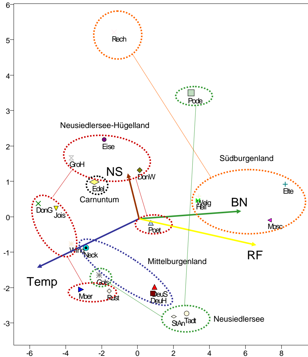
Abb. 5: Hauptkomponentenanalyse der Wetterdaten der Stationen. Ähnliche Daten bedingen einen geringeren Abstand der Standorte in der Grafik.
