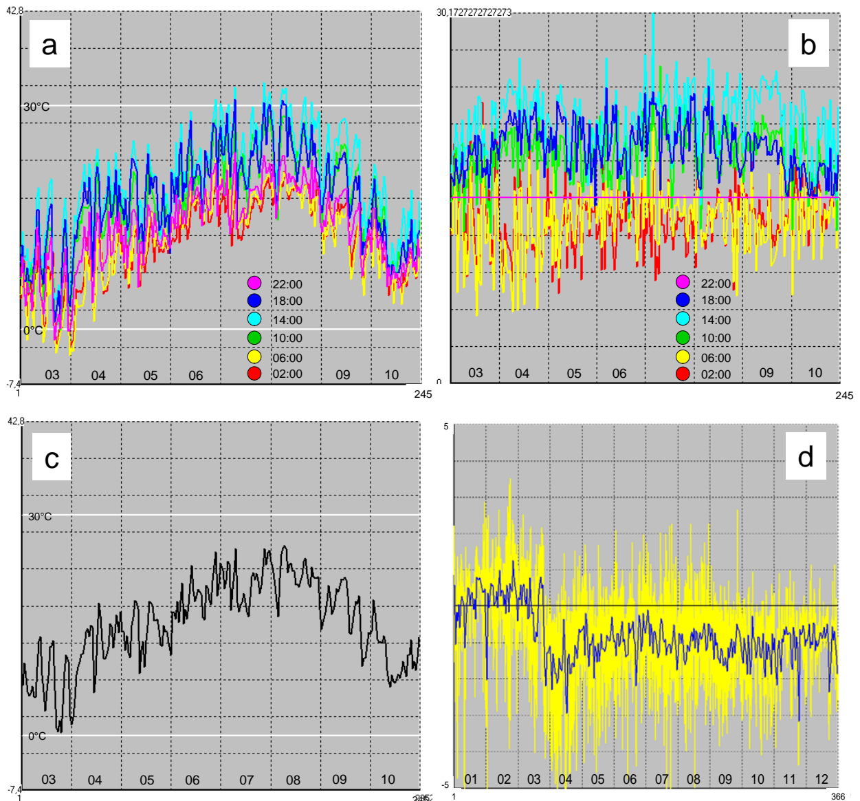
Abb. 1: Verschiedene Darstellungsformen der Lufttemperatur (in °C) für den Zeitbereich 01.03.2020 bis 31.10.2020 (a-c). Präsentiert ist der Mittelwert über alle Stationen. Abb. 1a: Lufttemperatur zu verschiedenen Tageszeiten. Abb. 1b: wie 1a, wobei allerdings die Abweichung von der Temperatur um 22 Uhr gezeigt wird. Abb. 1c stellt die mittlere Tagestemperatur dar und Abb. 1d die Abweichung der mittleren Tagestemperatur am Standort Podersdorf vom Mittelwert aller Standorte (blaue Linie). Gelb ist die Abweichung für jeden Messzeitpunkt (96 pro Tag) vom Mittelwert aller Standorte dargestellt. In Abb. 1d ist der Zeitbereich 01.01.2020 bis 31.12.2020 gezeigt.
